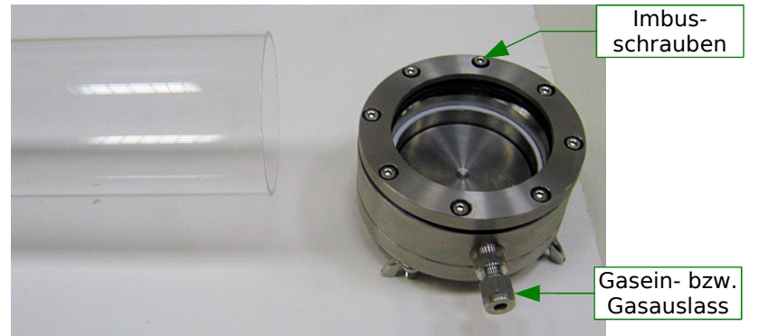
Abbildung 5: demontierter Endverschluss
